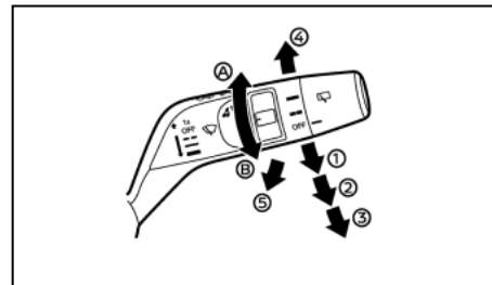
Τύπος A (χωρίς λειτουργία <AUTO>)
